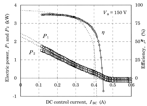
図7 入出力電力特性の計算結果と観測結果の比較
