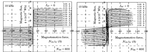
図4 ブリッジ結合磁路の磁束制御特性計算例
