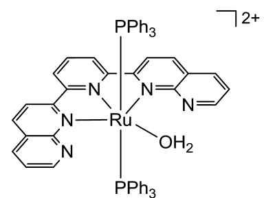
図2 本研究で用いたハイブリッド化合物の化学構造（PPh 3 ：トリフェニルホスフィン分子）
