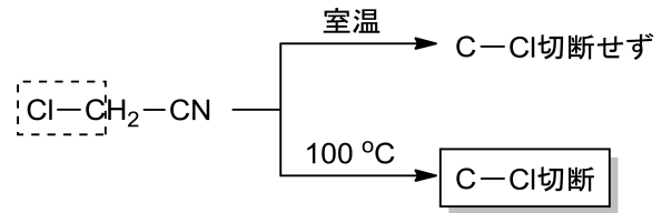
図4 クロロアセトニトリル分子中の炭素-塩素結合切断反応
