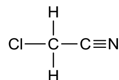
図3 クロロアセトニトリルの化学構造
