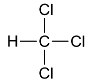
図1 クロロホルムの化学構造（C：炭素，Cl：塩素，H：水素）
